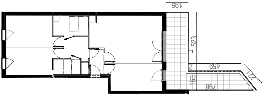
Plan des espaces extérieurs
